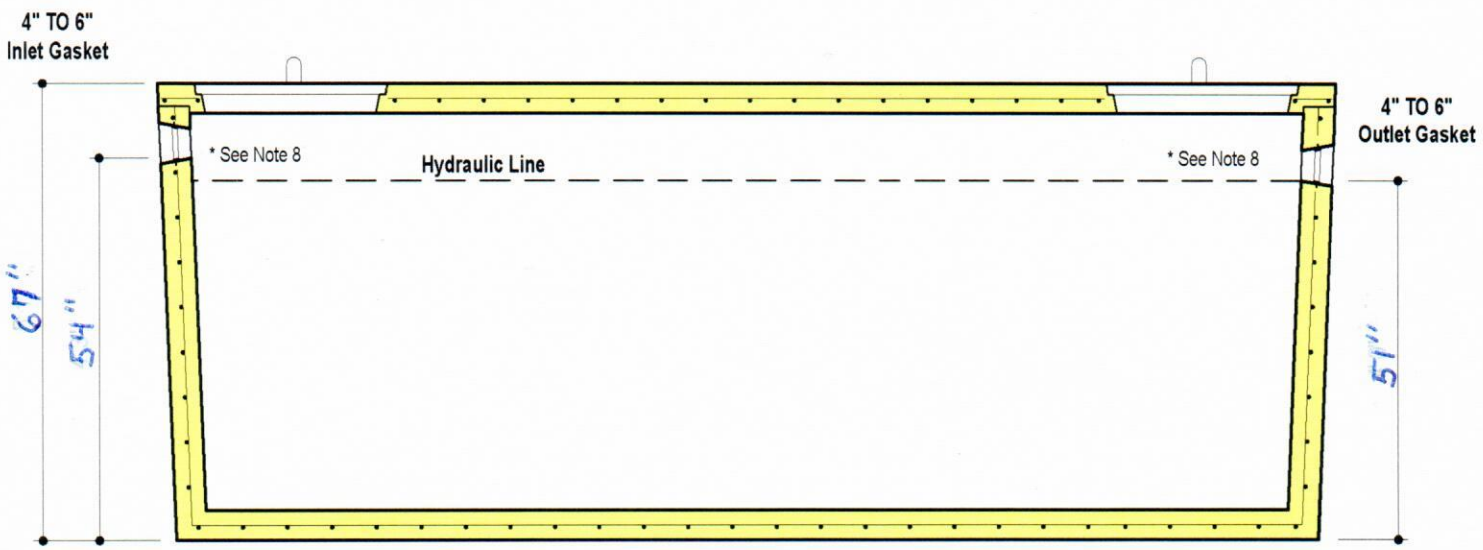
SECTION A-A
