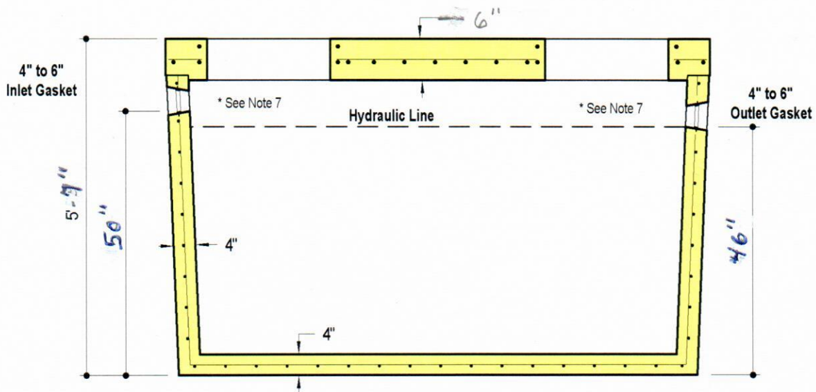
SECTION A-A
